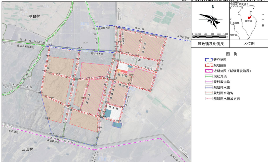
13-5 雨水设施规划图 (宣和片区)
