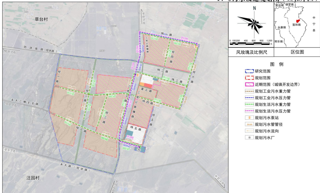
14-5 污水设施规划图 (宣和片区)
