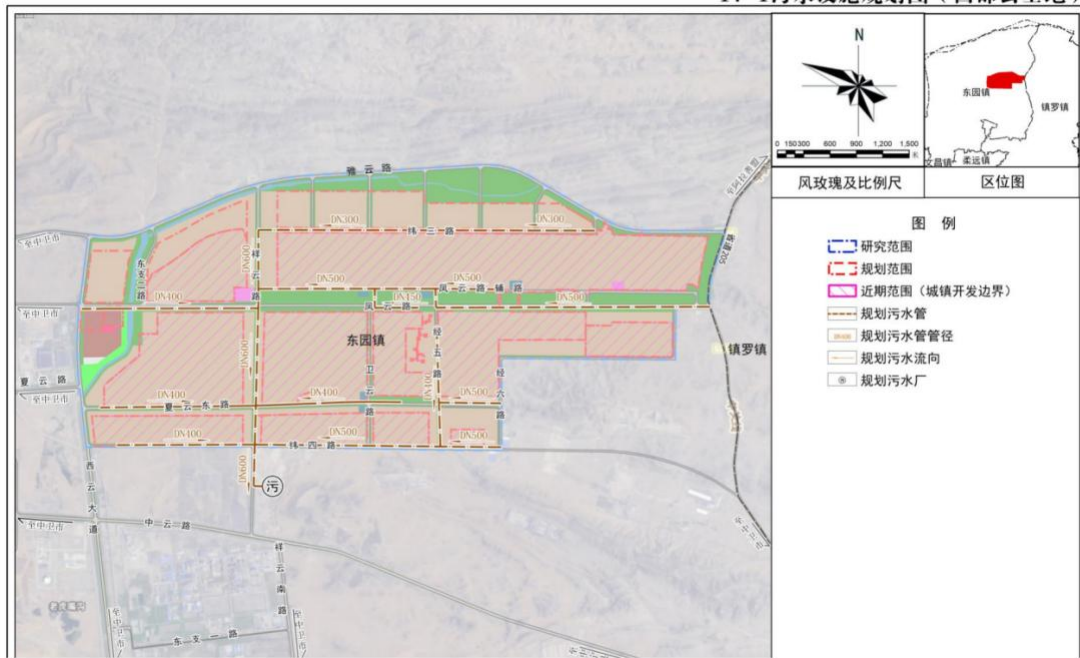
14-5 污水设施规划图 (宣和片区)
