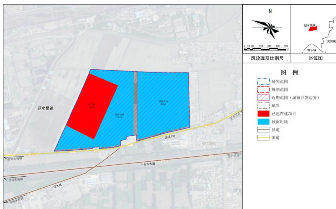
图 4-7 迎水桥片区用地布局图
