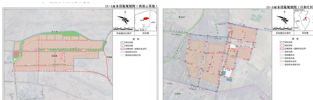
图 6-10 雨水设施规划图
