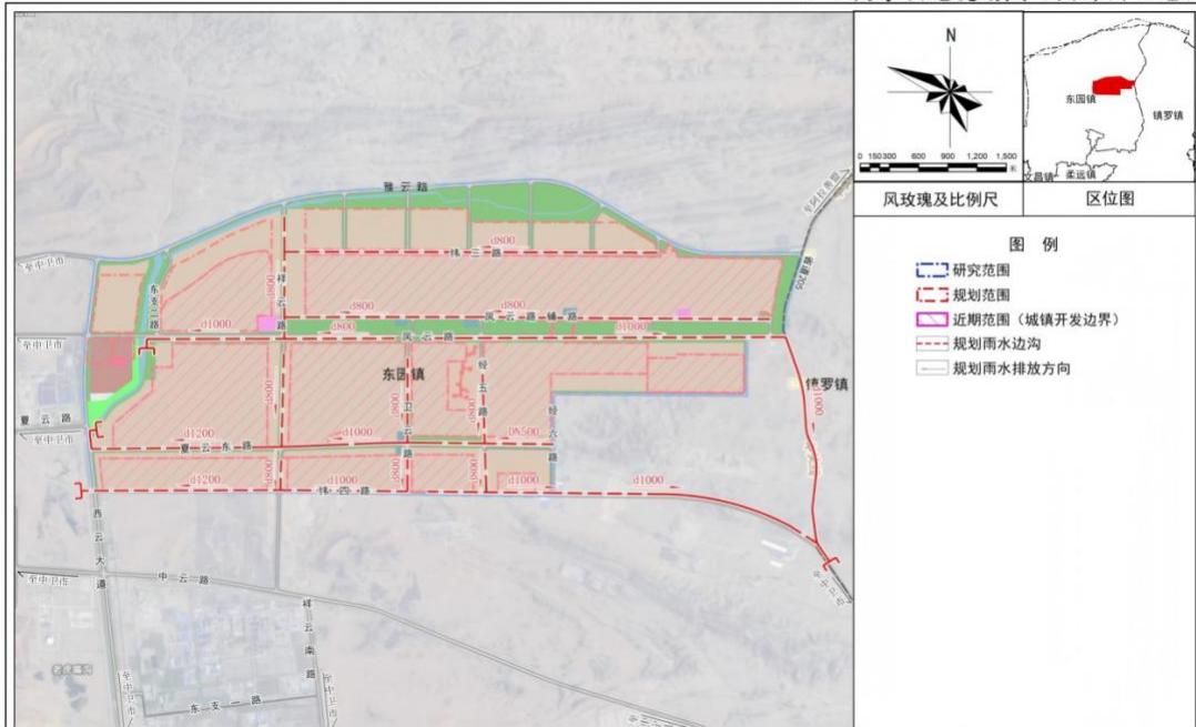
13-5 雨水设施规划图 (宣和片区)
