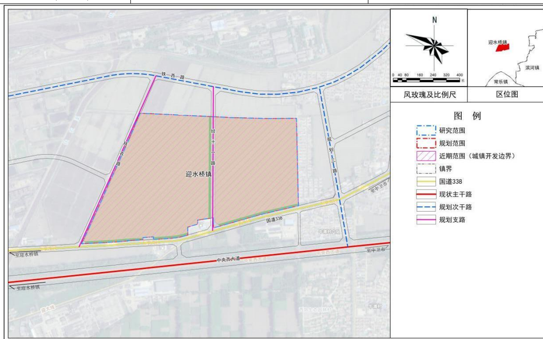
图 6-4 道路交通规划图（迎水桥片区）
